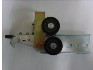
2) LG-OTIS INTERLOCK SILA1
