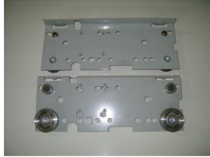
2) 기전 L2 모델 카 측
