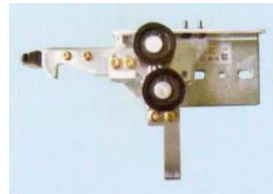
6) LG-OTIS INTERLOCK DEVICE
