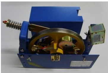
9. 가바나 LG-OTIS (PCD240, 305)
