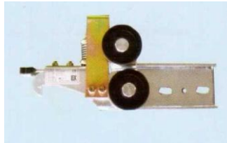
5) LG-OTIS INTERLOCK DEVICE
