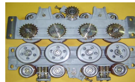
12. LG-OTIS HR 구동장치
