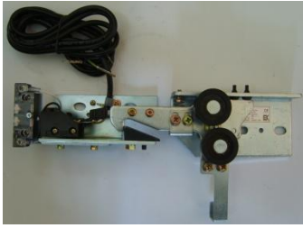
1) LG-OTIS SBD 시그마 인터록세트
