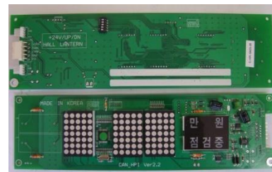
11) 중소업체, 표시기, CAN-HPI
