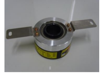
4) 티센동양 엔코더 DY100-1024DO
