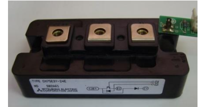
4) IGBT 모듈 CM75E3Y-24E
