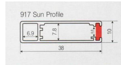
8) WECO, 도어빔센서 전망용(내광식),SUN
