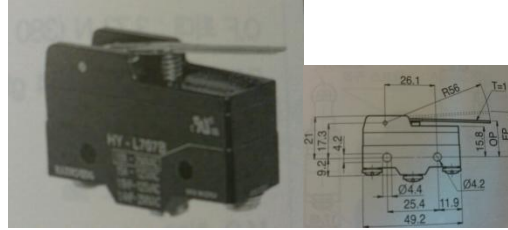
2) 마이크로스위치 중 레버형
