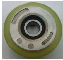
2. 현대 스텝롤러 D76*W20*B6203
