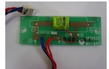
12) LG-OTIS PCB 용 배터리
