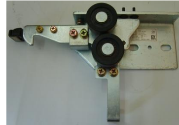
3) LG-OTIS SBD 시그마 인터록 가동자
