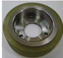
6. LG기전 J형 ES HR구동롤러 D130,W33
