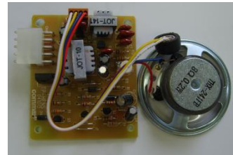
6) 인터폰 자기 분리형
