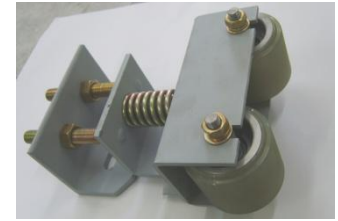
4. LG-OTIS HR 가압롤러
