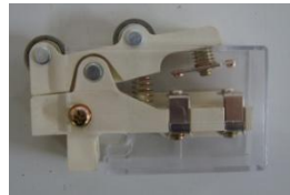
7) LG-OTIS 도어스위치 A, B접점
