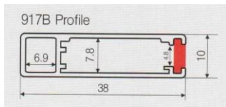
5) WECO, 도어빔센서 양측고정, 917B
