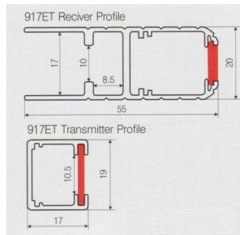
6) WECO, 도어빔센서 한쪽가동, 917ET
