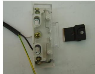
6) OTIS 인터록 은접점세트
