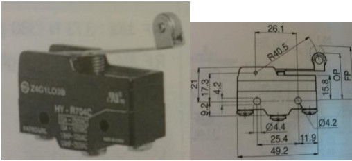
5) 마이크로스위치 힌지롤러 레버형
